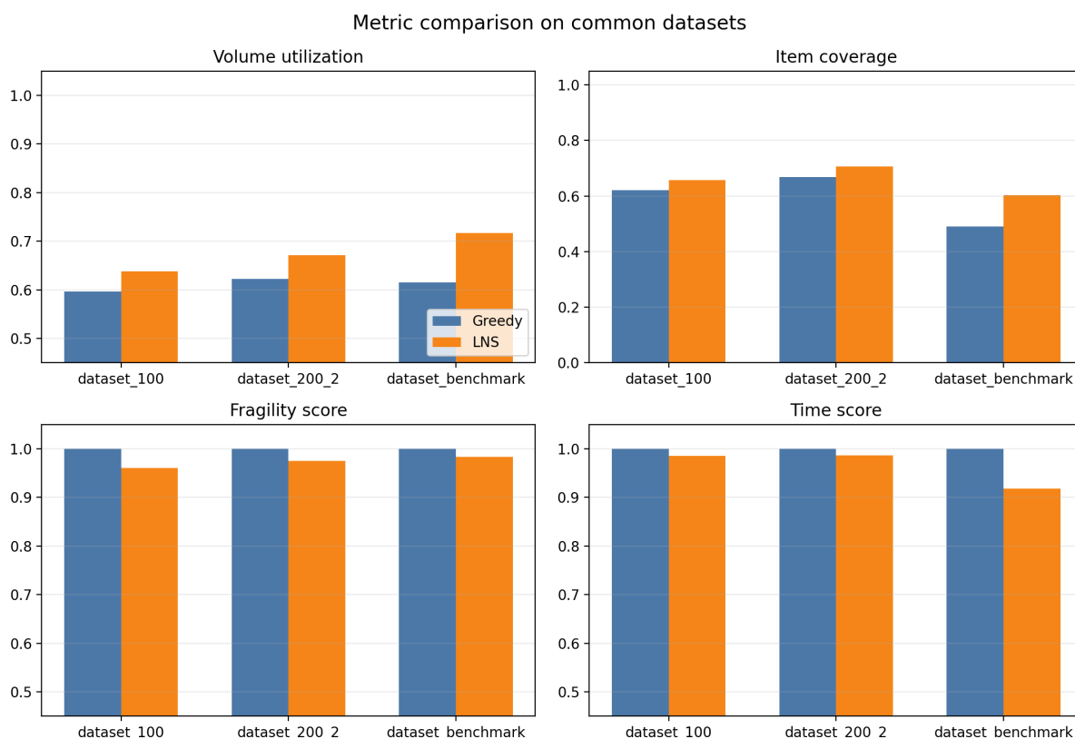
Рисунок 7 – Сравнение компонент метрики для LNS и greedy
