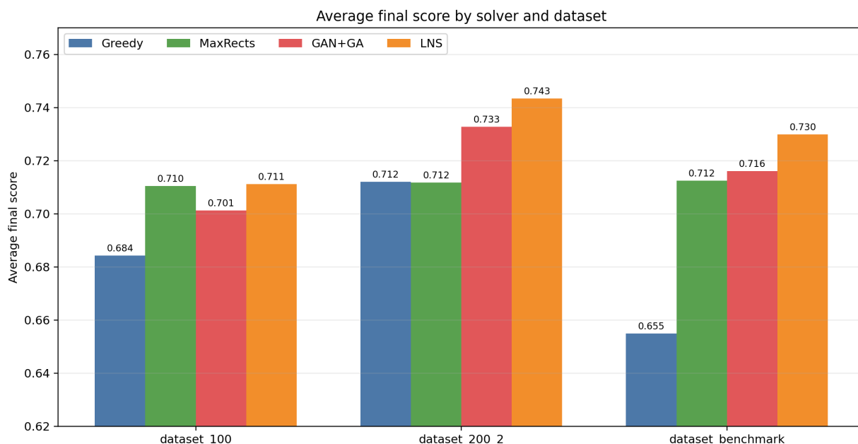
Рисунок 4 – Средний итоговый score по решателям и датасетам
