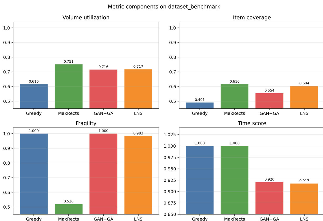
Рисунок 5 – Компоненты score на контрольном наборе
