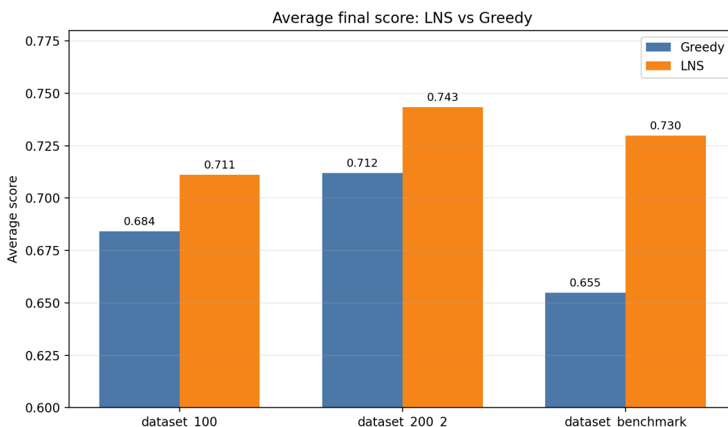
Рисунок 6 – Сравнение среднего score для LNS и greedy
